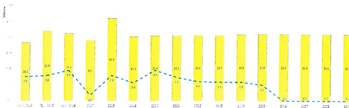
Wykres 3 Nadwyżka operacyjna i rozchody w latach 2014-2029 dla Gminy Suchy Las (w mln PLN)
